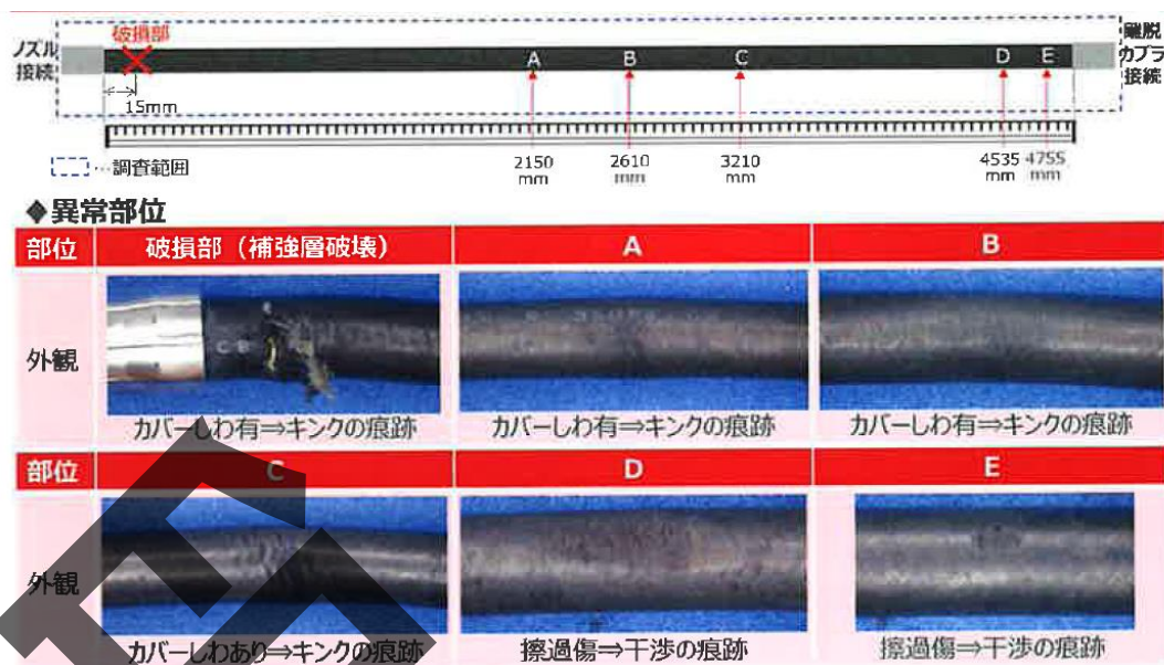
図 C.4 ディスペンサーに設置されたフレキシブルホースの異常の例 (2020 年度事故概要報告 2019-378)
